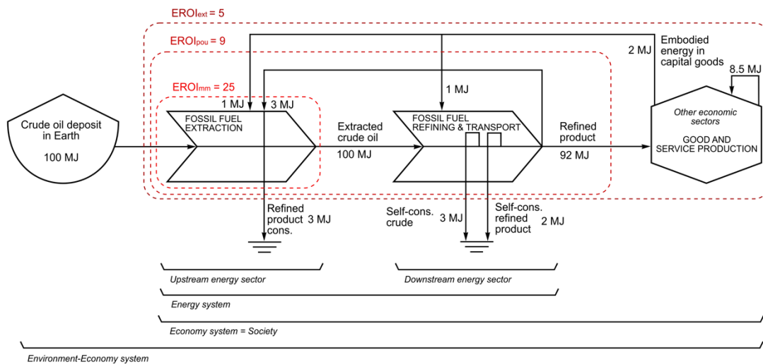
Figure 3. Frontières de différents EROI associés à l'exemple de l'extraction et du raffinage de 100 MJ de pétrole brut. Source : auteur.
